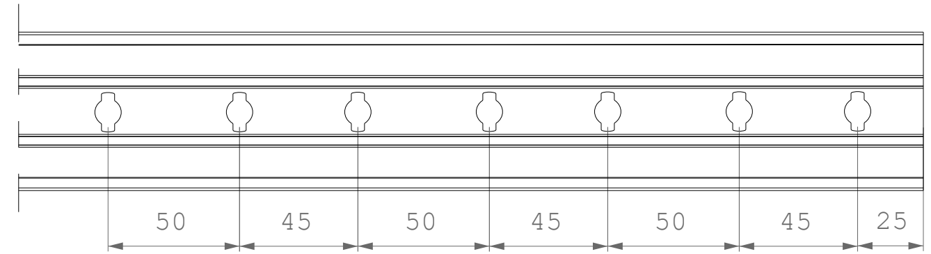
Detail 1:2
